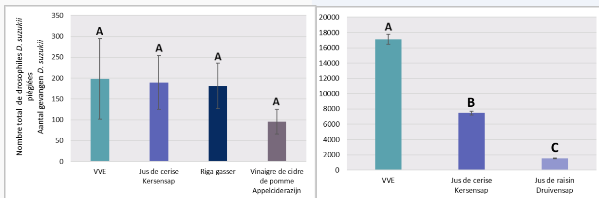
Figure 1 : Nombre de drosophiles D. suzukii piégées en 2020, en Belgique (gauche) et en France (droite). Des lettres différentes indiquent les différences statistiques.
